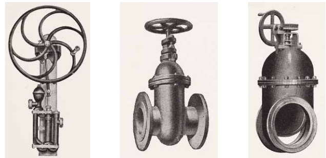
Bomba aspirant i vàlvules de comporta. Catàleg de Bombas GEYDA. Carlos Gens, S.L. Imprés al setembre de 1947.
